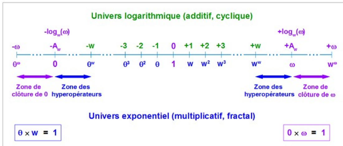
Structure de l'ensemble R_\omega des nombres omégaréels
