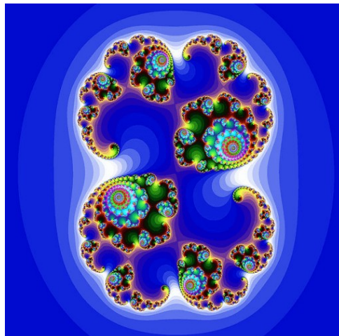
Deux symétries centrales ou radiaires.
